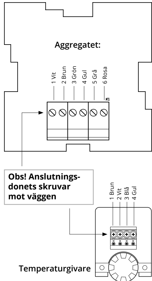
Koppling av kretskort i styrenheten
