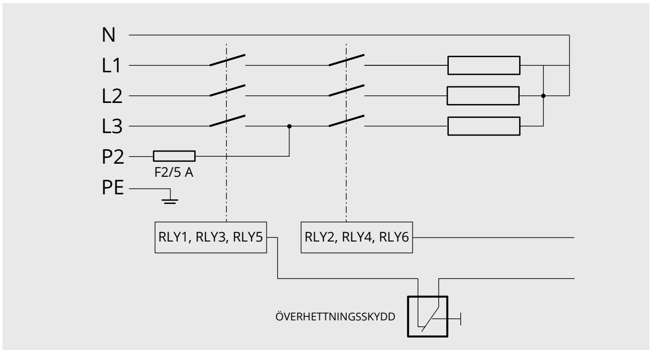
Koppling av kretskort i aggregatet
