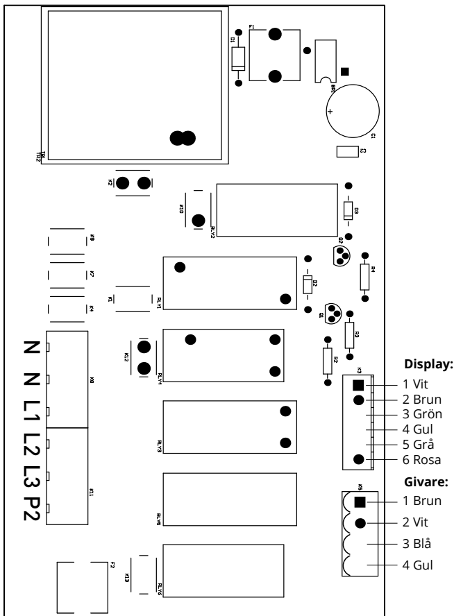
Koppling av kretskort i aggregatet
